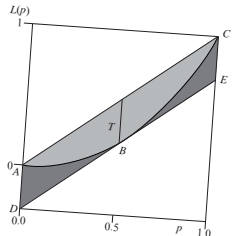
Rys. 1.8. Ilustracja indeksu polaryzacji Wolfsonego Źródło: opracowanie własne
